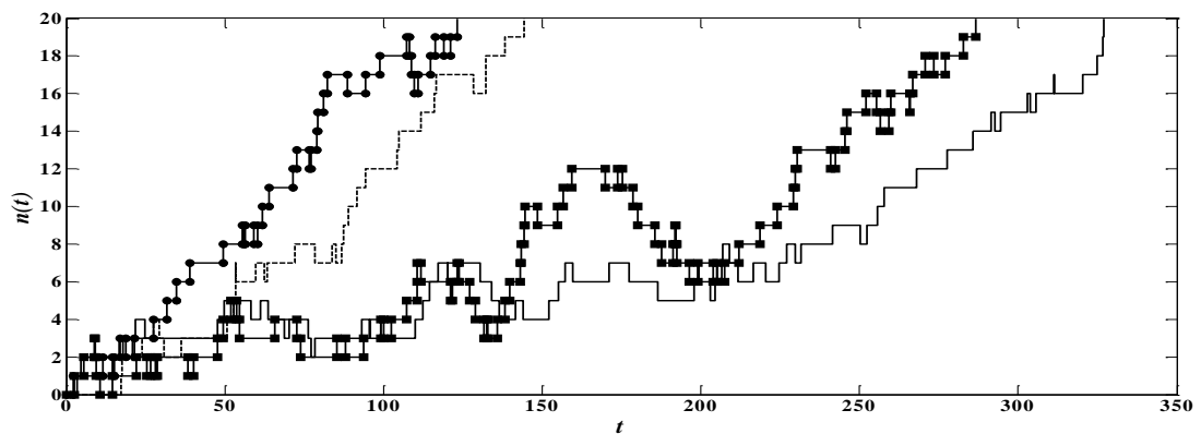
Рис. 4. Пример четырех реализаций накопления числа дефектов n(t)
