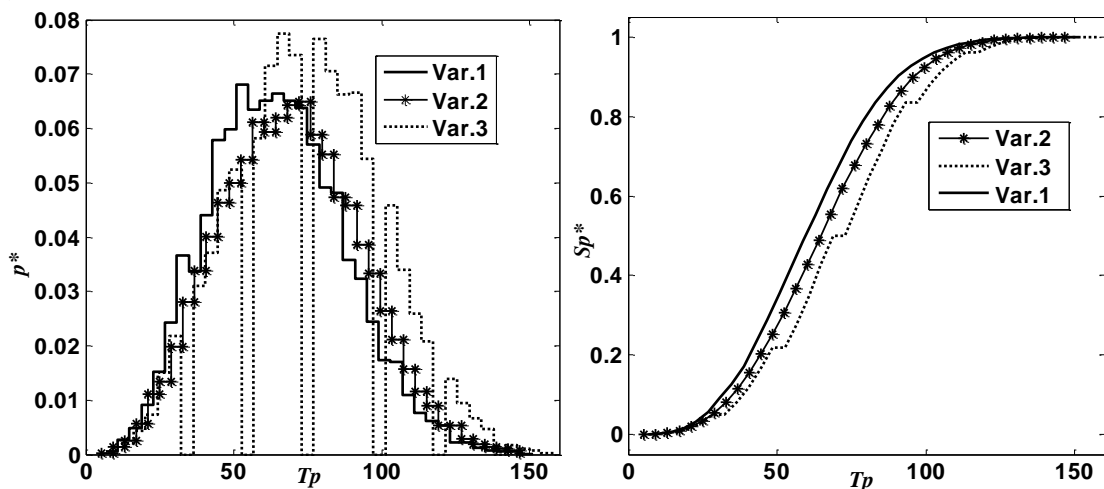
Рис. 7. Оценки функций плотности вероятностей p^* и интегральных функций распределения Sp^* для Tr
