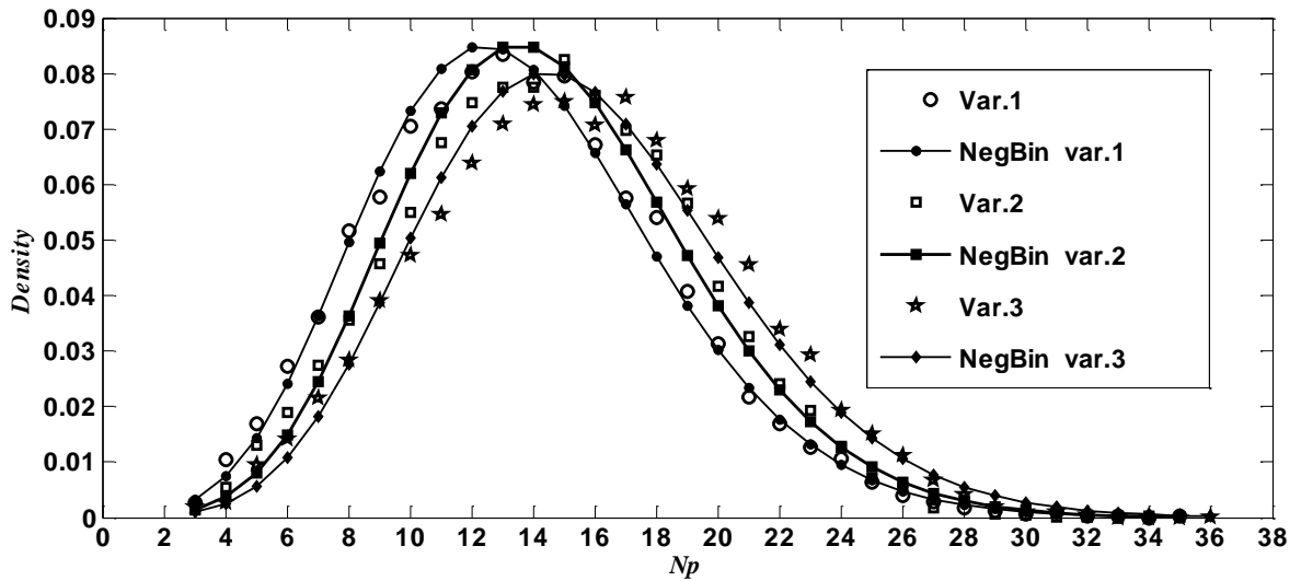
Рис. 10. Распределения NegBin для трех вариантов модели
